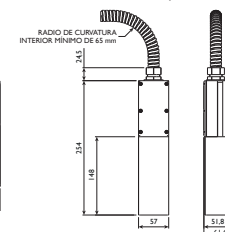
Cabezal de impresión Duo
